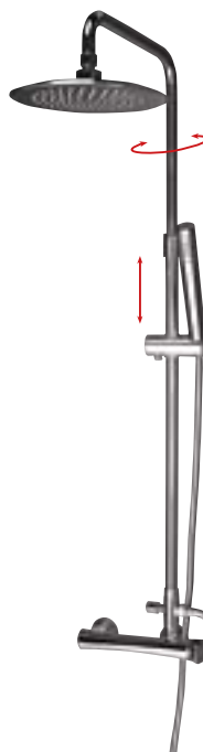
990E Zuhanyoszlop csapterlep nélkül, zuhanszettel, Ø fejuhany: 200 mm, állítható magasság: 830-1280 mm 127.990,-
