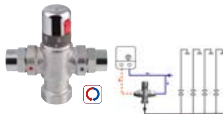
TMTCOM Termostatikus keverőszelep 4-8 fogyasztóig, 20-50 °C, F1"x F3/4", visszacapó szeleppel, szűrővel 49.990,-
